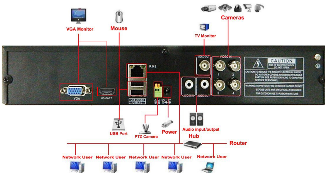
Rys. 2. 1 Pełny diagram połączeń
